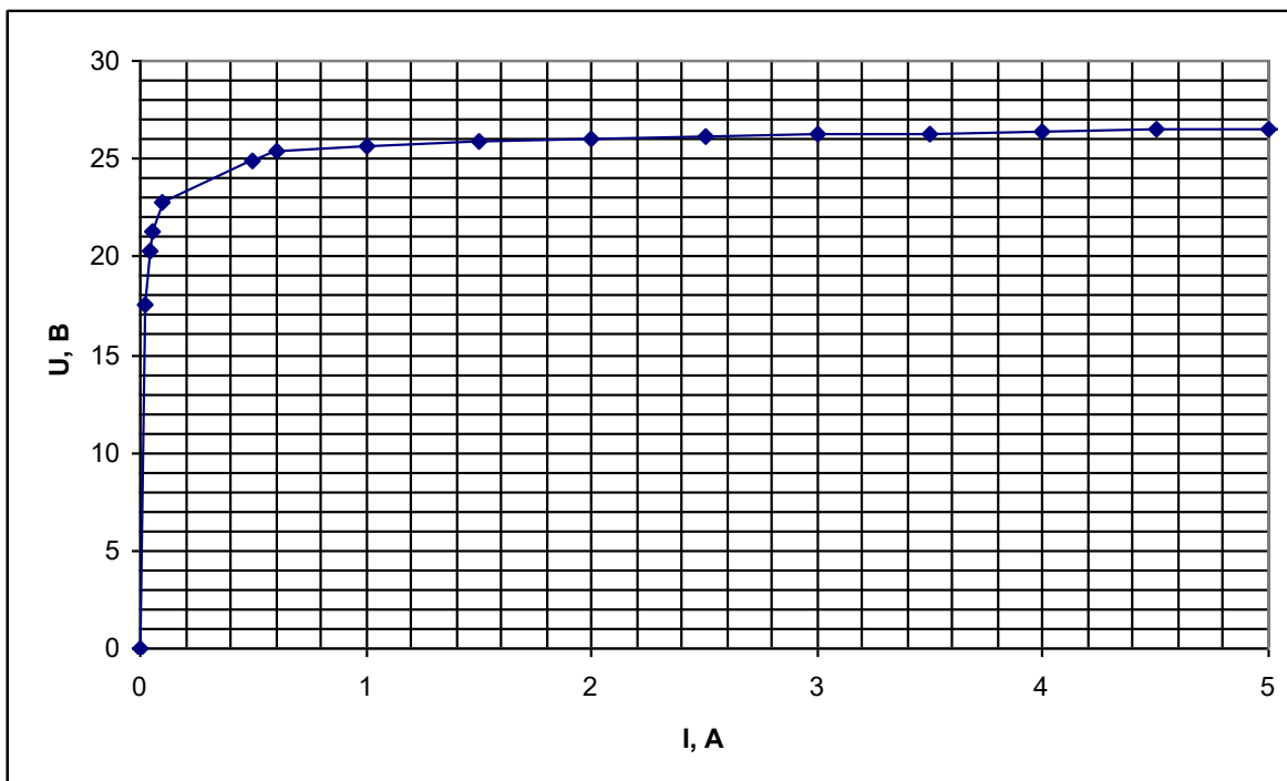
ВАХ вторичной обмотки для измерения с КТ 0,5; 0,5S; 0,2; 0,2S , номинальной нагрузкой 10 \text{ В} \cdot \text{А} и K_{\text{БНОМ}}=10 трансформаторов с первичным током 2000 \text{ А} . Сопротивление обмотки постоянному току – 0,19 \text{ Ом} .
