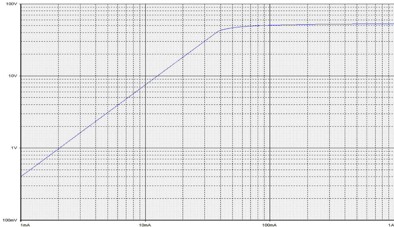
ВАХ вторичной обмотки для защиты с КТ 10Р, номинальной нагрузкой 15 \text{ В} \cdot \text{А} и K_{\text{НОМ}}=10 трансформаторов с первичным током 1500 \text{ А} . Сопротивление обмотки постоянному току – 0,23 \text{ Ом} .
